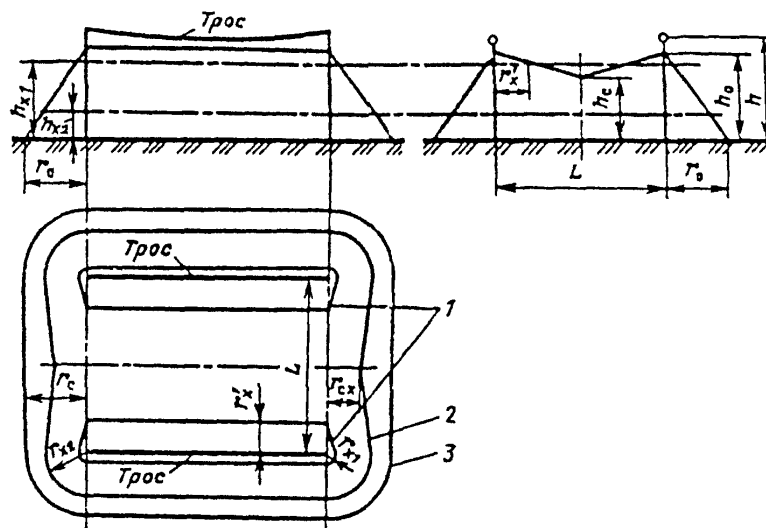
Рис. ПЗ.6. Зона защиты двойного тросового молниеотвода. Обозначения те же, что и на рис. ПЗ.2
