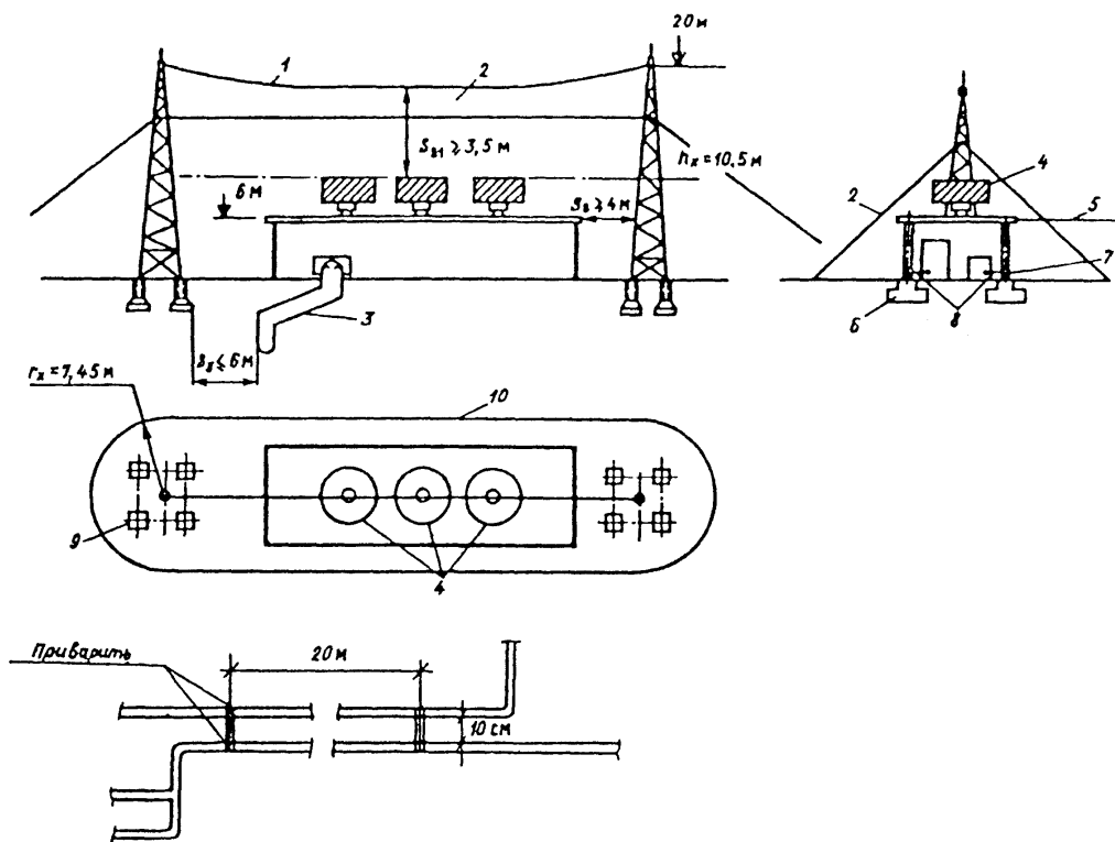
Рис. П4.3. Молниезащита здания I категории отдельно стоящим тросовым молниеотводом ( \rho = 300 \text{ Ом} \cdot \text{м} ,
