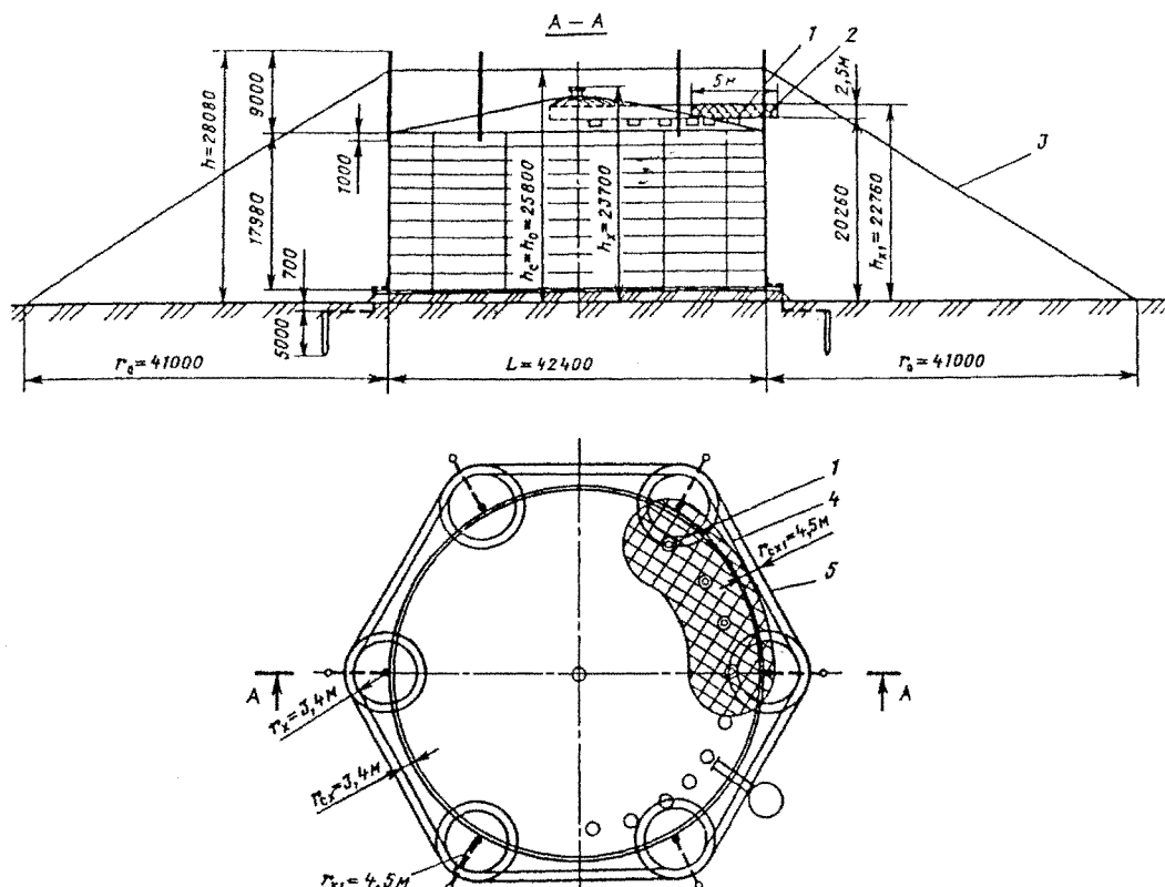
Рис. П4.7. Молниезащита металлического резервуара вместимостью 20 тыс. м 3 со сферической крышей: 1 - дыхательный клапан; 2 - область выброса газов взрывоопасной концентрации; 3 - граница зоны защиты; 4 - зона защиты на высоте h_x = 23,7 м; 5 - то же, на высоте h_x = 22,76 м
