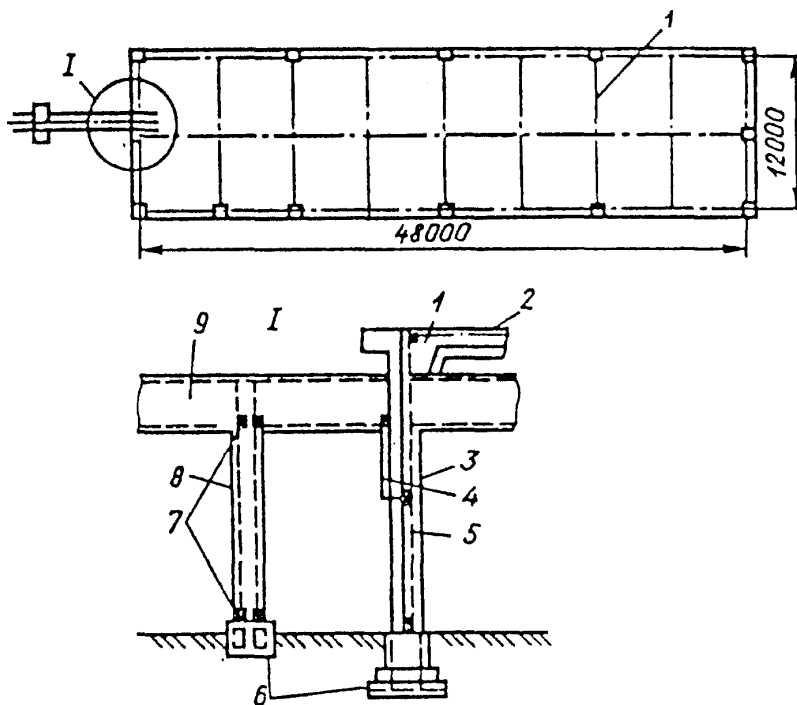
Рис. П4.4. Молниезащита здания II категории сеткой, уложенной на кровлю под гидроизоляцию:
