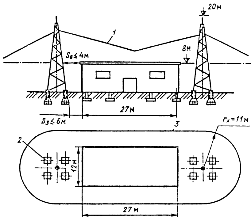
Рис. П4.2. Молниезащита здания I категории отдельно стоящим двойным стержневым молниеотводом ( \rho = 300 \text{ Ом} \cdot \text{м} ,
