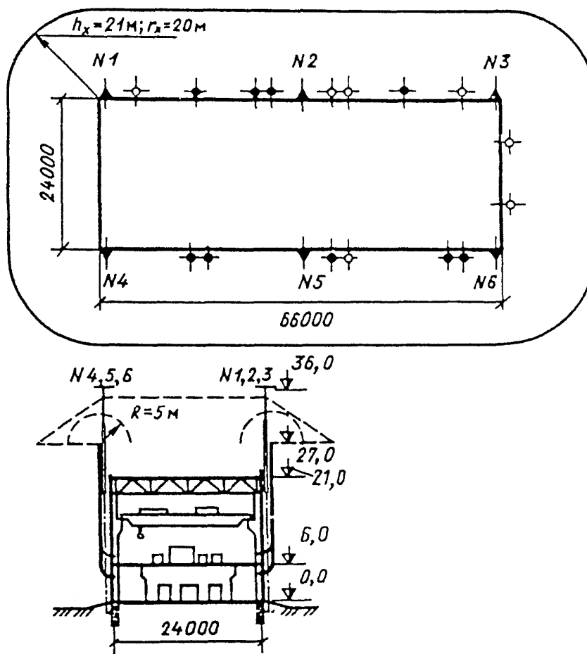
Рис. П4.6. План цеха компрессии азотоводородной смеси (относится к взрывоопасным с зоной класса В-Ia); Условные обозначения: ▲ - стержневой молниеотвод (N 1 - 6); —, —, — - токоотводящая металлическая полоса; ○ - газоотводные трубы для отвода в атмосферу газов невзрывоопасной концентрации; ● - то же, взрывоопасной концентрации
